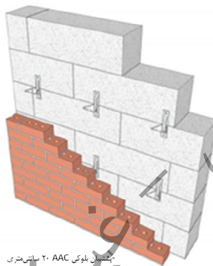
شکل ۴-۵- اتصال نمای آجری به دیوار بلوک AAC
