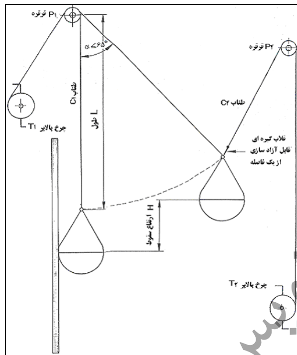
شکل ۳-۵- set up انجام آزمایش ضربه جسم نرم سنگین
