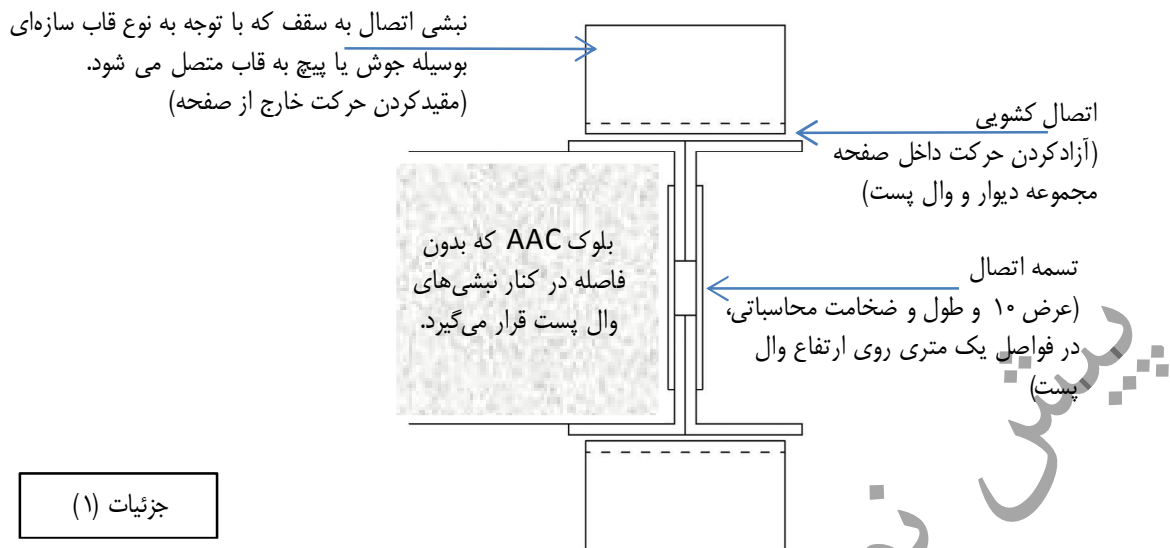
شکل ۴-۱۲- تامین آزادی حرکت جانبی برای مجموعه دیوار و وادار
