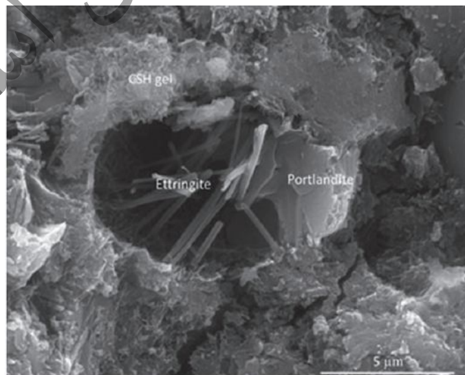
شکل ۳-۱- تصویر میکروسکوپی هیدرات‌های سیمان در دمای عادی
