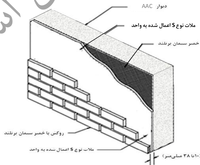
شکل ۵-۶- نمای چسبانده شده به دیوار پشتیبان AAC
