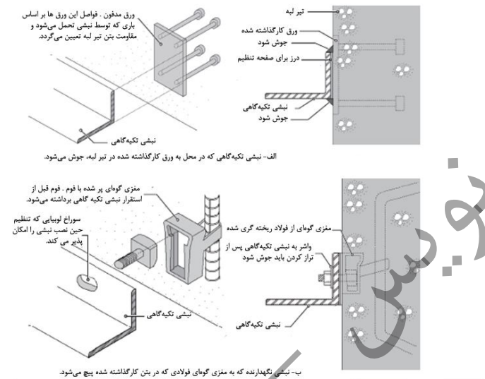
شکل ۵-۱۷- جزئیات اجرایی اتصال نبشی تکیه‌گاهی به دیوار پشتیبان
