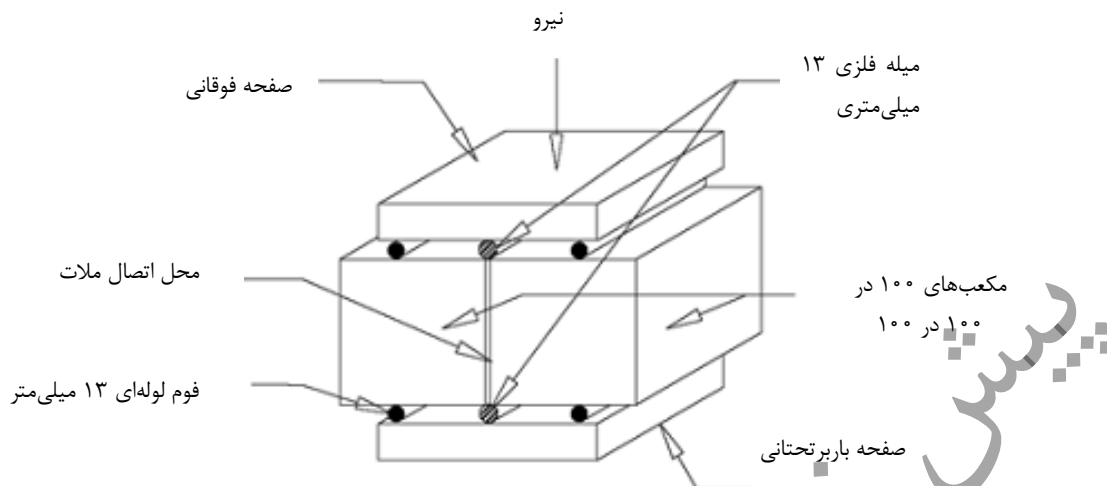
شکل ۲-۲- آزمون مقاومت گسیختگی کششی
