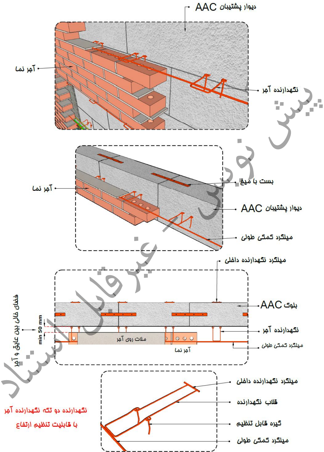
شکل ۵-۱۶- جزئیات مهار نما به کمک دیوار AAC
