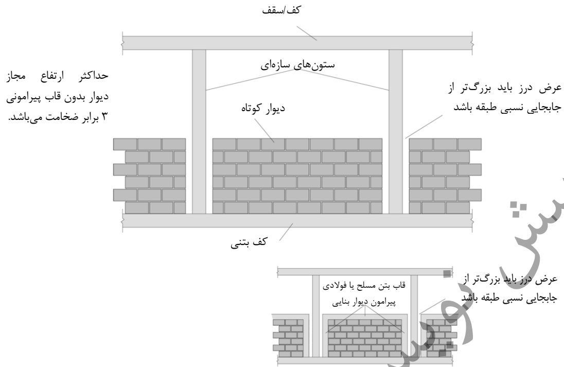
شکل ۳-۱- پارتیشن کوتاه
