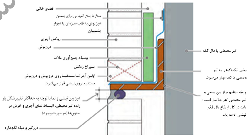
شکل ۵-۱۰- جزئیات شماتیک نبشی تکیه‌گاهی
