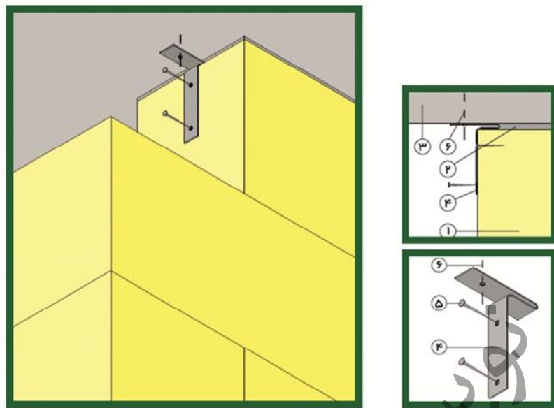
۱- دیوار AAC
